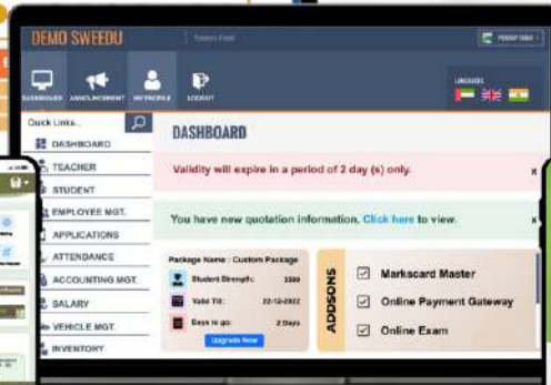
Web Panel
